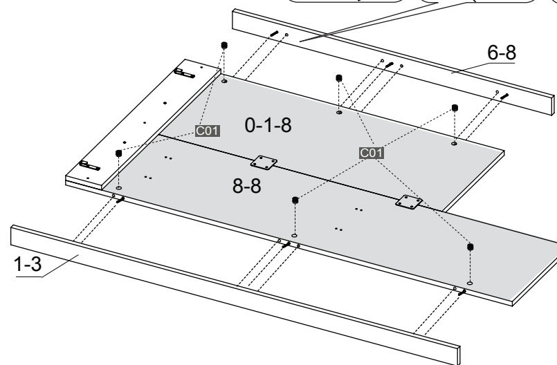
Стяжка эксцентриковая
