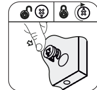
Стяжка эксцентриковая
