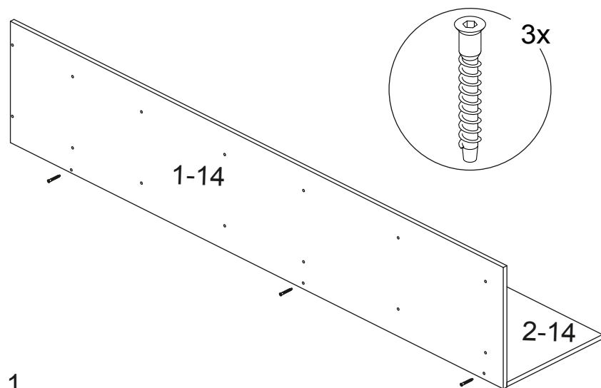
2.1 Сборка стеллажа при установке его с левой стороны шкафов (рис. 1)
