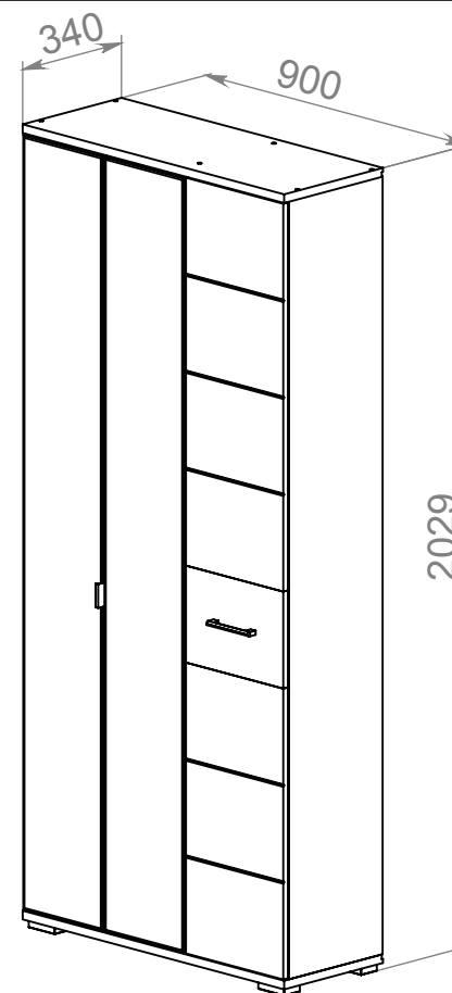
Шкаф ПМ-293.01.00.000
