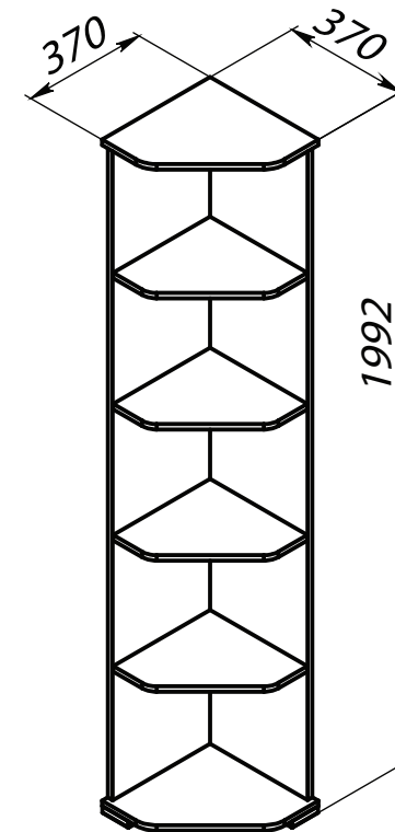
Стеллаж ПМ-229.14.00.000
