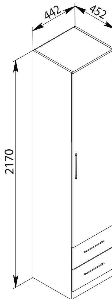
Шкаф для белья комбинированный ПМ-277.02.00.000
