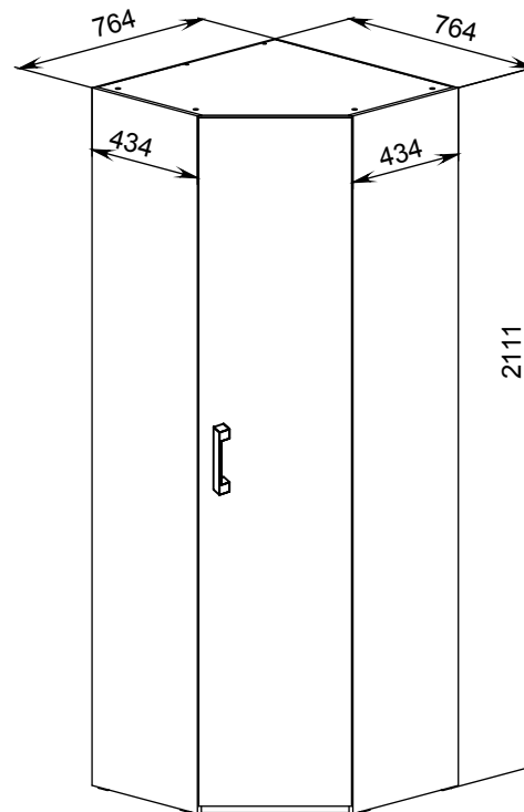
Исполнение правое
