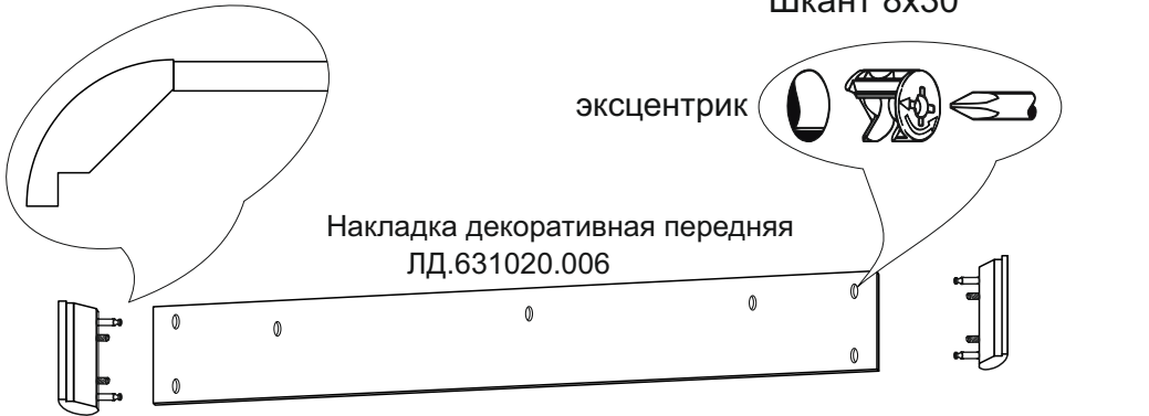
Шкант 8x30
