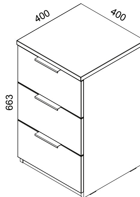
Тумба с тремя ящиками ПМ-298.05.00.000
