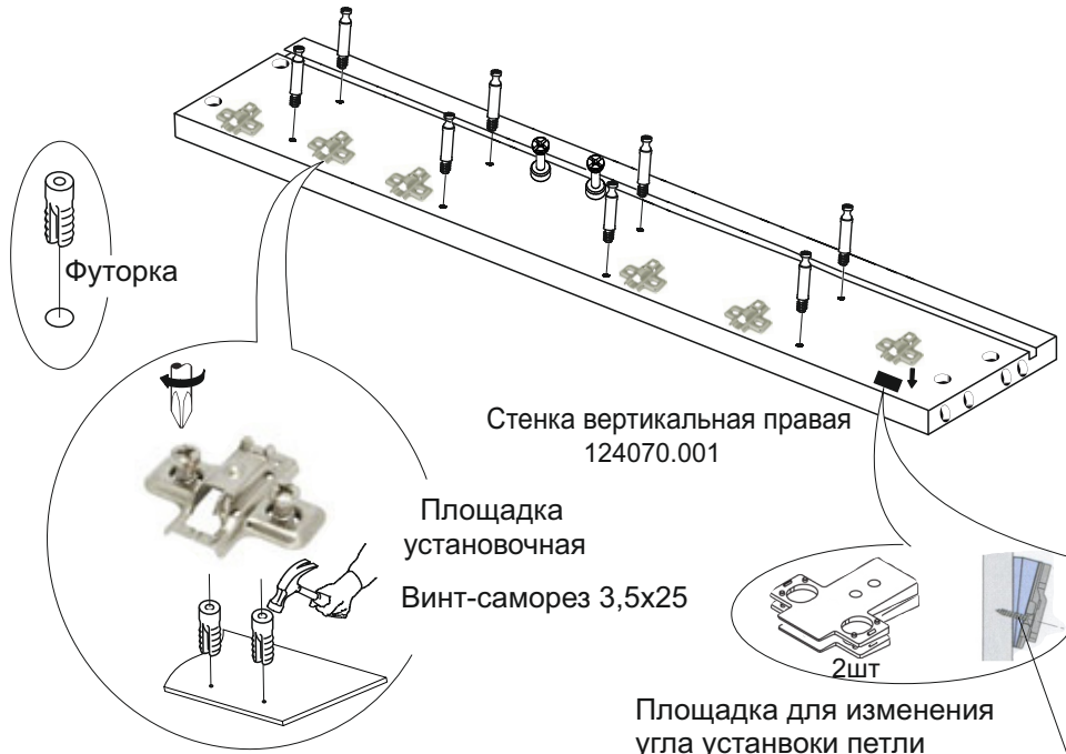
Винт-саморез 3,5x25
