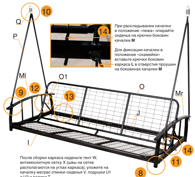
11 Крепление опоры спинки к боковине качалки M Болт М8х40 Шайба 8 Гайка М8 Колпачок на М8
