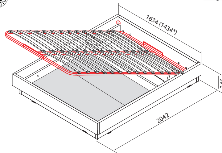
Каркас кровати с подъемным механизмом: ТД-193.01.02 - 1600x2000 ТД-193.02.02* - 1400x2000
