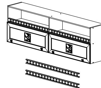
Балюстрада для шкафа навесного ПМ-300.16.00.000
