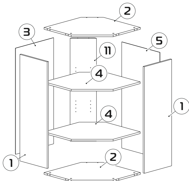
б - модуль высотой 960 мм
