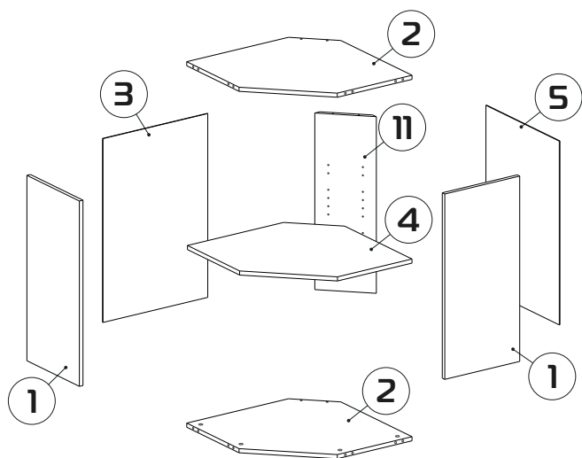
а- модуль высотой 720 мм
