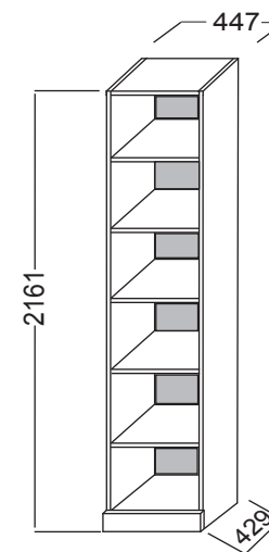
Каркас шкафа для белья ПМ-235.21.00.000 ТД 235.07.21
