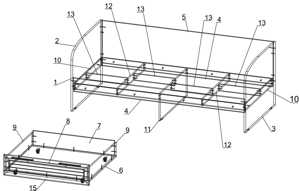
Перечень деталей
