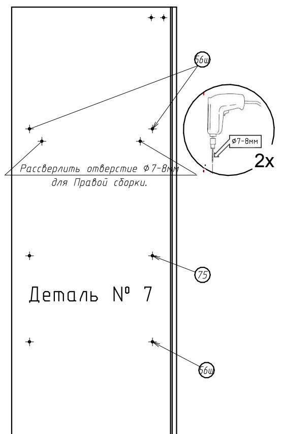
Правая сборка :
