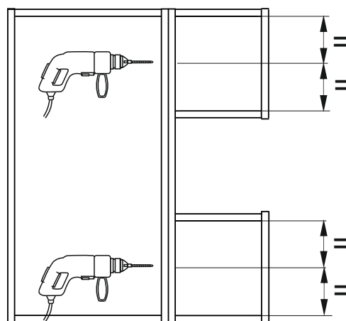
Соединение с навесными и напольными каркасами
