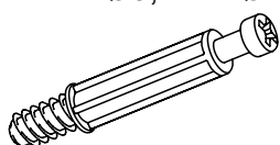
Шток эксцентриковой стяжки \varnothing 6,2 \times 11 \varnothing 7 \times 30
